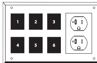
MPOC-3XUAC MPOC-3XU plus 110V/20A AC Duplex Outlet & 6 Connectors
