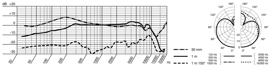
Risposta in frequenza e diagramma polare: HSD 171, HSD 271
