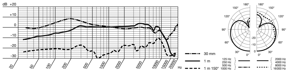
Réponse en fréquence et diagramme polaire pour HSD 171, HSD 271
