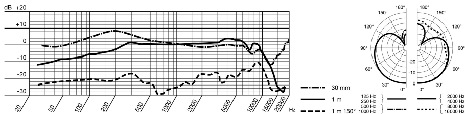
Resposta de frequência e diagrama polar: HSD 171, HSD 271
