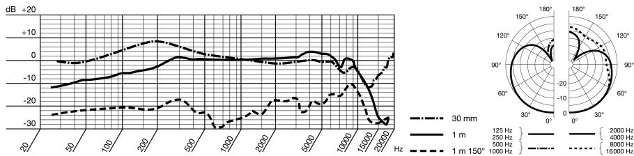
Respuesta de frecuencia y diagrama polar: HSD 171, HSD 271
