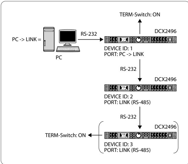
Fig. 4.30: PC -> LINK mode
