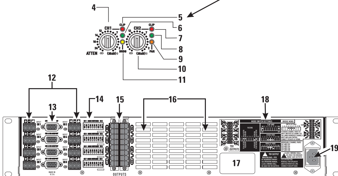
后面板
