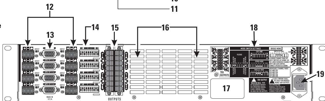
Rückplatte
