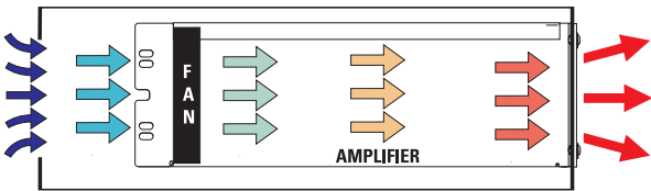
QSC 放大器内气流：冷却风扇将冷空气吹入放大器后部。热风从放大器前盖流出。
