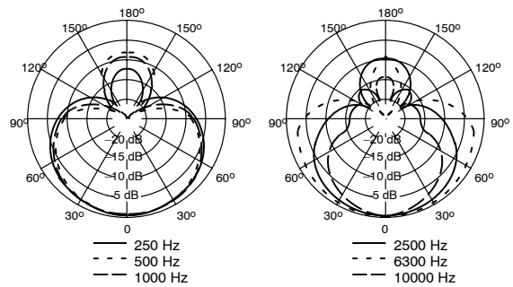
TIPICI DIAGRAMMI POLARI FIGURA 3
