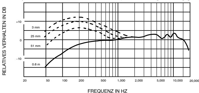
TYPISCHES FREQUENZVERHALTEN ABILDUNG 2
