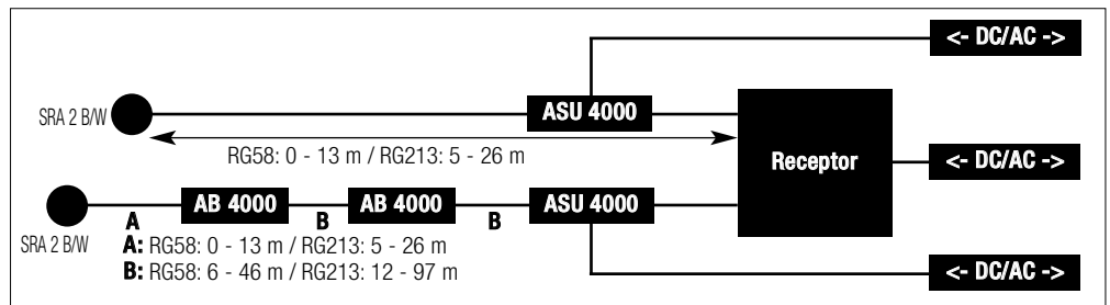
Fig. 7: Cableado de un sistema monocal con antenas activas y tramos de cable de longitudes diferentes.
