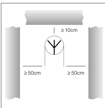
Fig. 4: Mindestabstand von ebenen Flächen
