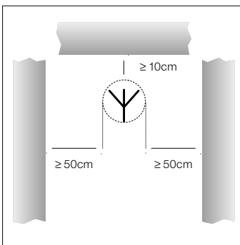
Fig. 4 : Distance minimum d'une surface plane
