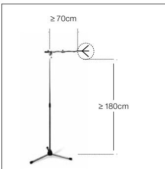
Fig. 3: Antenne auf Bodenstativ montiert
