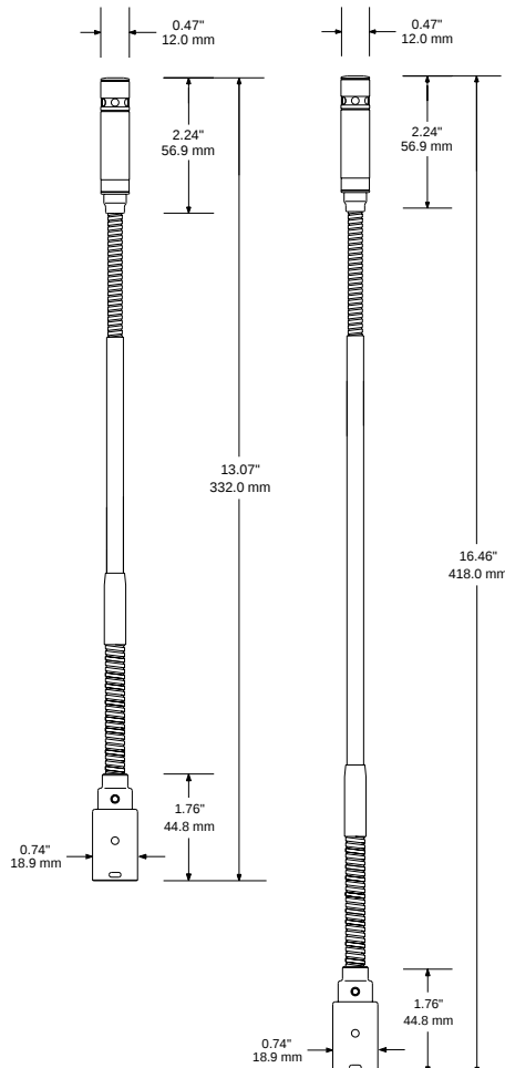
PRO 49Q Dimensions
