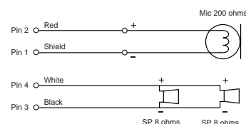
CC-60 WIRING
