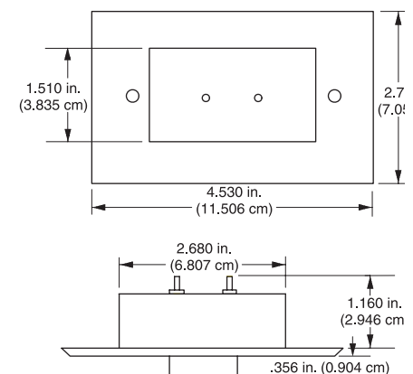
Fig. 2. Dimensions
