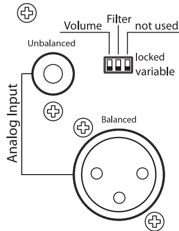
Rückseitige Anschlüsse &amp; DIP-Schalter
