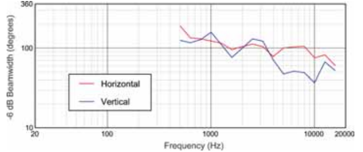
Beamwidth
