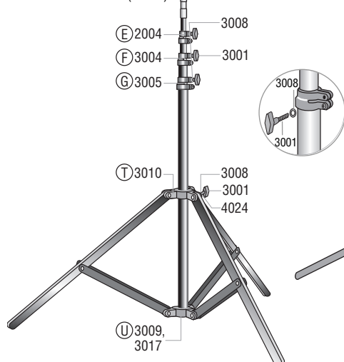
KS Jr Stand (KSJR)
