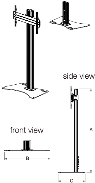
DS-600SP-AL
