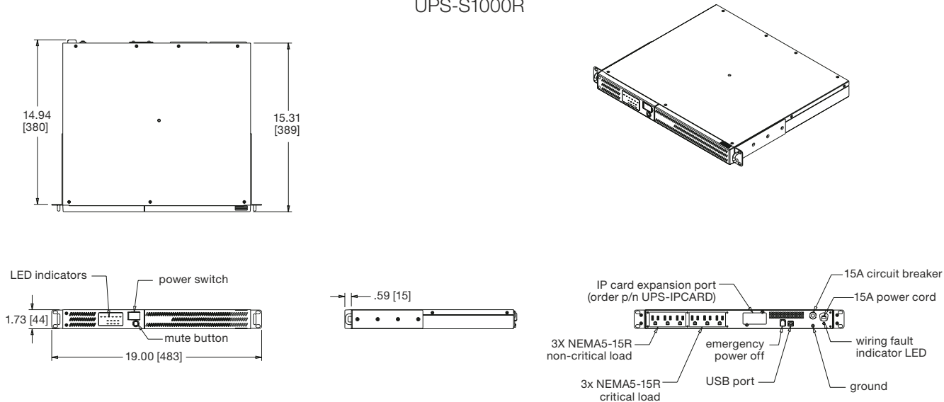
UPS-S1000R
