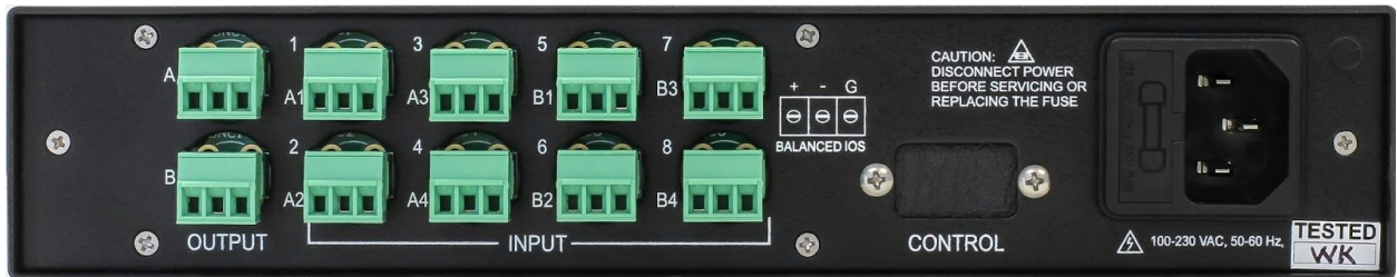
POD10A/110 REAR
