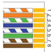
T-568B
