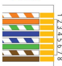
T-568B
