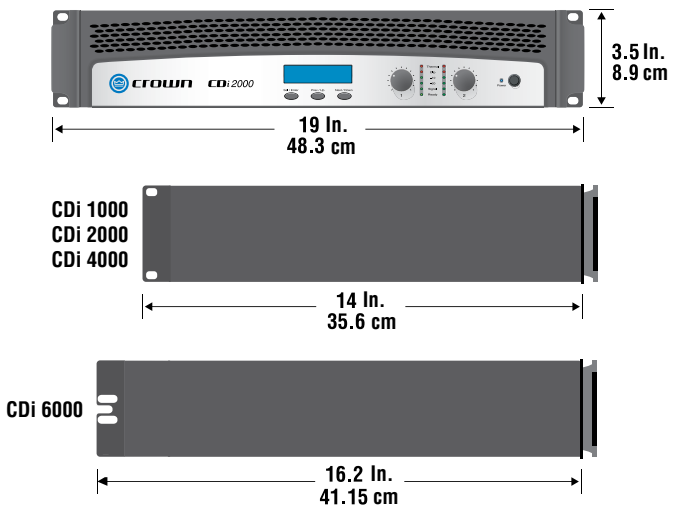
Abb. 2.1 Abmessungen
