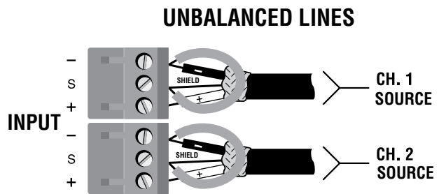
Abb. 2.3 Symmetrischer (oben) und unsymmetrischer (unten)
