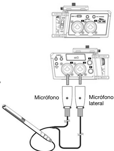
Figura 2: Conecte los micrófonos central y lateral a las entradas.
