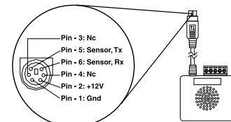
Рисунок 1: Разъем PS/2 датчика EnviroSense
