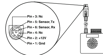
Figure 1 : Connecteur PS/2 EnviroSense
