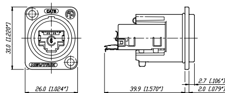
NE8FDY-C6
