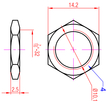
NUT
